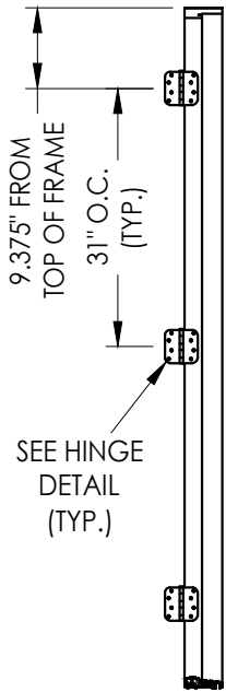
HINGE JAMB
